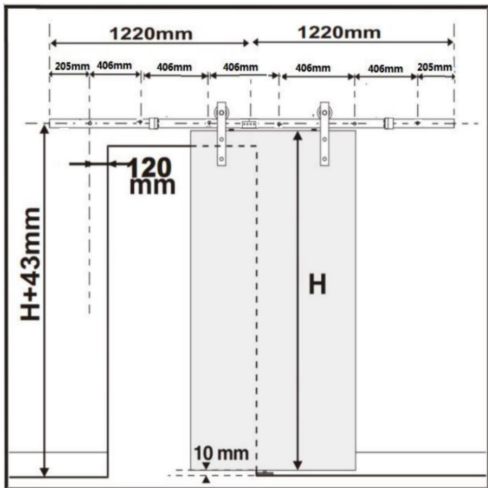
8ft Pojedyncze drzwi
