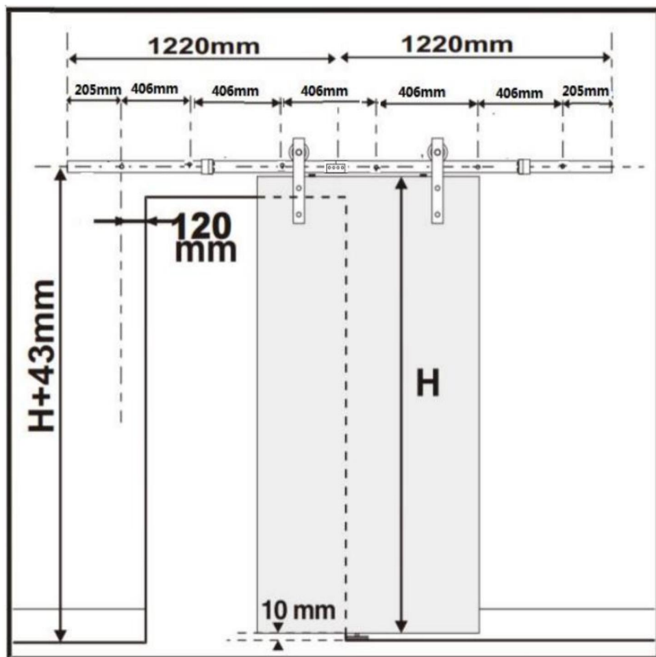
Porta singola da 8 piedi
