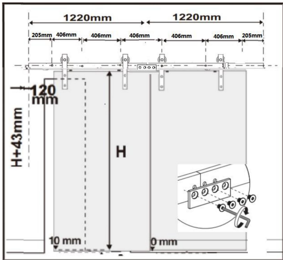
Puerta doble de 8 pies
