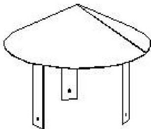
A) Osłona: \varnothing 135 \times 108 \text{ mm}
