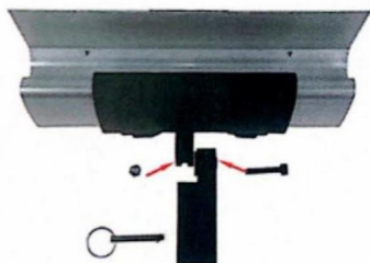
3. Fissare il gruppo vite.
