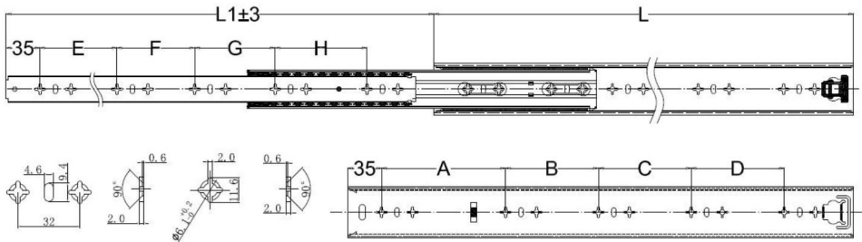
Schéma de perçage d'installation 5301/5301Z (unités : mm)
