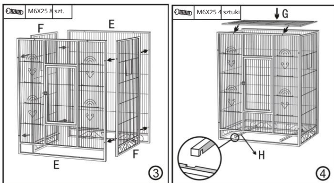
3. Wyjmij siatkę żelazną i złóż ją
