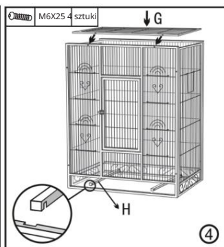
4. Załóż górną siatkę i suport.
