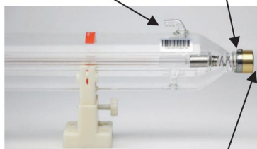
Uscita acqua (rivolta verso l'alto) Elettrodo negativo (-)
