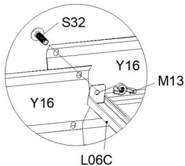
3. Połączenie korbowodu z prostą płytą.
