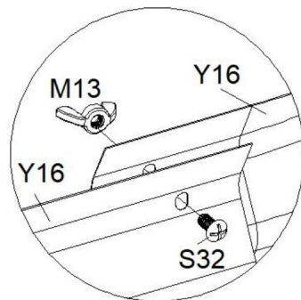
2. Połączenie prostych płyt.
