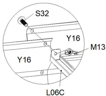
3. La connexion d'une bielle à une plaque droite.
