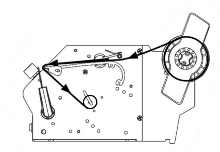
Etikettenpapierroute
