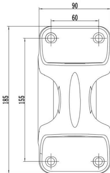
Gat voor kunststof wandbeugel
