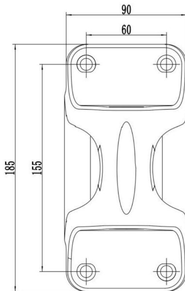
Otwór na plastikowy uchwyt ścienny
